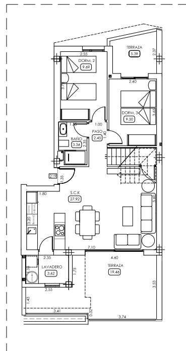
PLANTA 2
