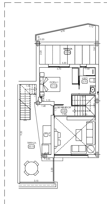
PLANTA ÁTICO
