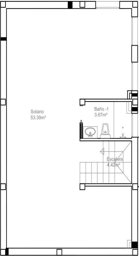
PLANTA SÓTANO 61,48m 2
