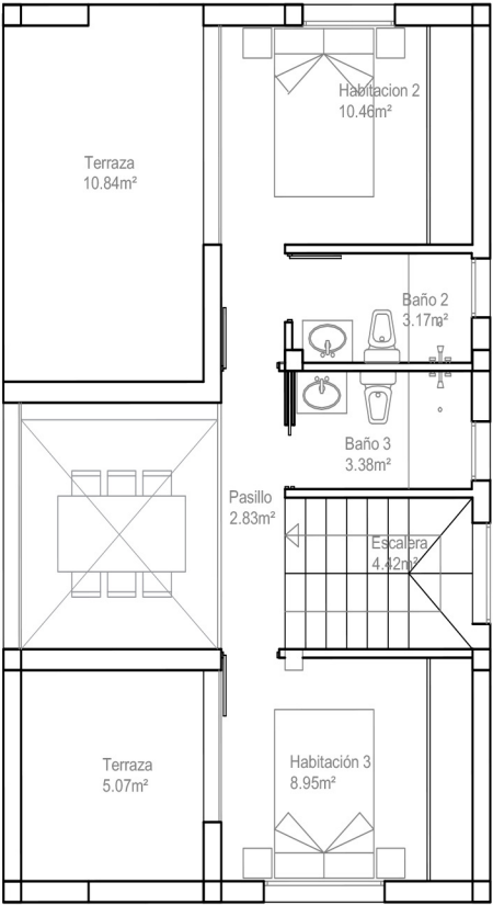
PLANTA PRIMERA 49,12m 2
