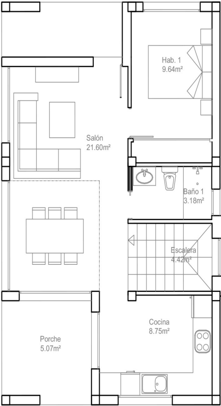
PLANTA BAJA 52,66m 2
